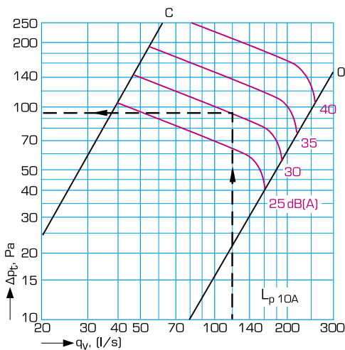
EHC-800-150
