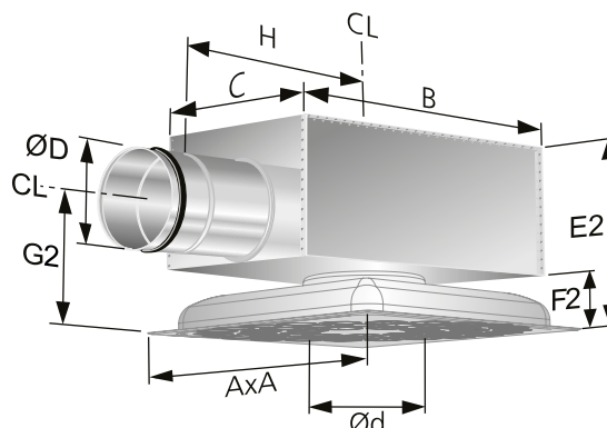
Figur 7. COLIBRI Ceiling med ALS. Låg bygghöjd.
