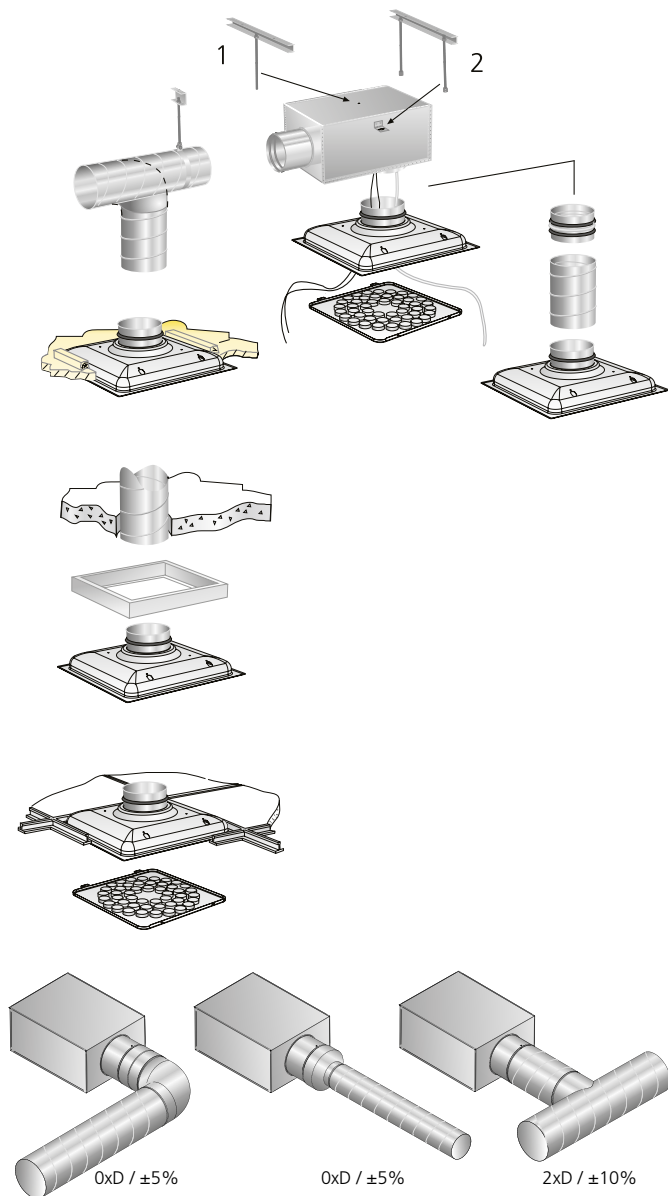
Figur 2. Monteringsalternativ.
