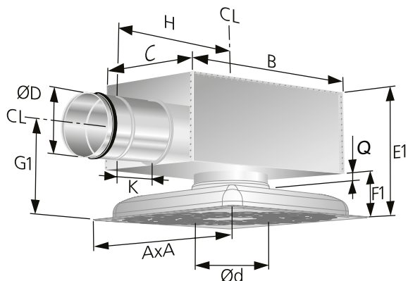
Figur 5. COLIBRI Ceiling med ALS. CL = Centrumlinje.
