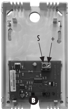
%RH-anturin elektroniikkakortti
