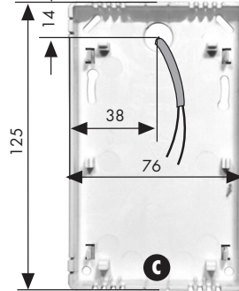
%RH-anturin pohjalevy
